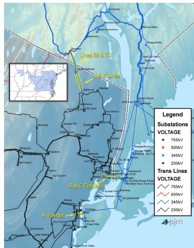
Figure E-1 Con Edison wheel
